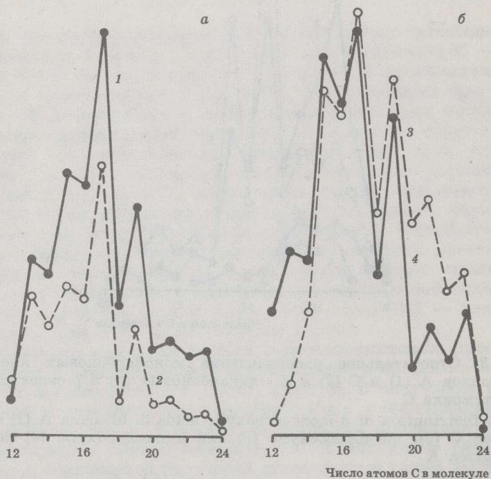
Рис. 4. Относительное распределение: а — «симметричных» (1) и метилалканонов (2); б — n -алкилбензолов (3) и n -алкилциклогексанов (4) битумоида А
